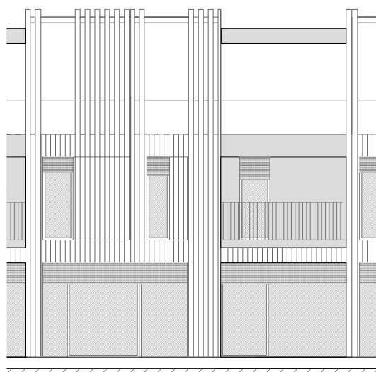
PROSPETTO INTERNO 1:100
