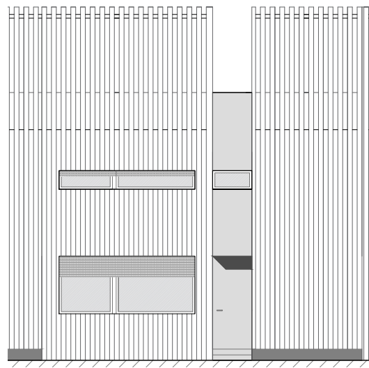
PROSPETTO ESTERNO 1:100
